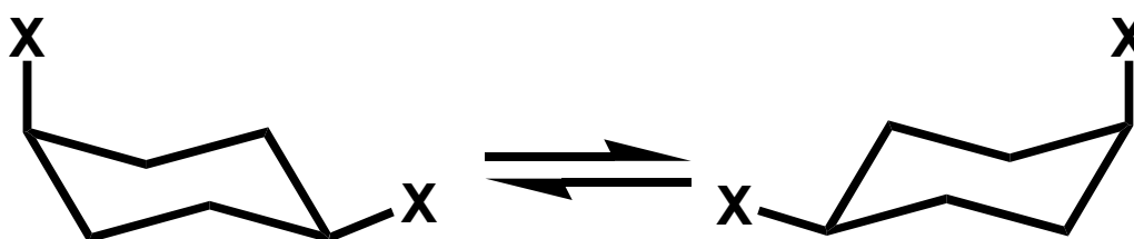
Cisz -1,4-di-X-ciklohexán konformerjei
