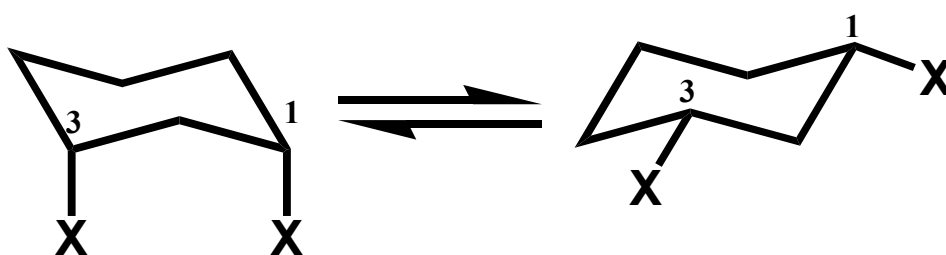
Cisz -1,3-di-X-ciklohexán konformerjei
