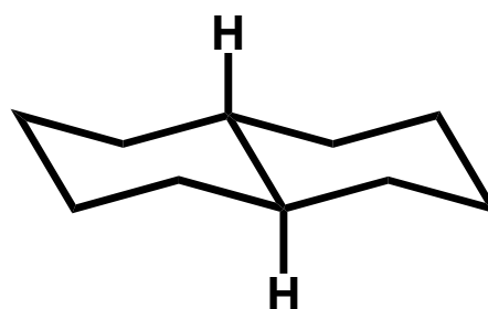
transz -dekalin
