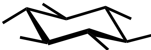
Ekvatoriális kötések
