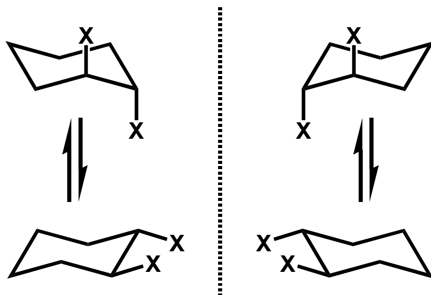
Trans -1,2-di-X-ciklohexánok enantiomerjeinek konformációs viszonyai
