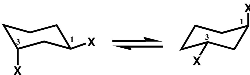
Trans -1,3-di-X-ciklohexán konformerjei
