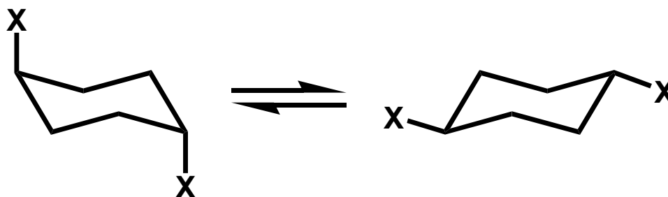
Transz -1,4-di-X-ciklohexán konformerjei
