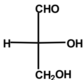
D-Glicerinaldehid
